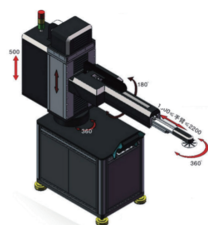
摆臂机器人
